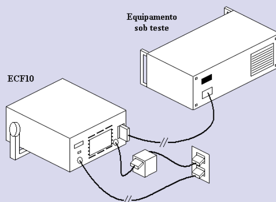
Ensaio de corrente de fuga para o terra com o ECF10.
